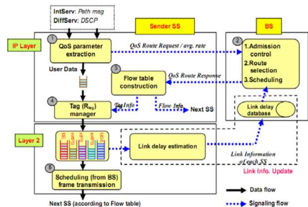
Fig. 2 QoS framework
